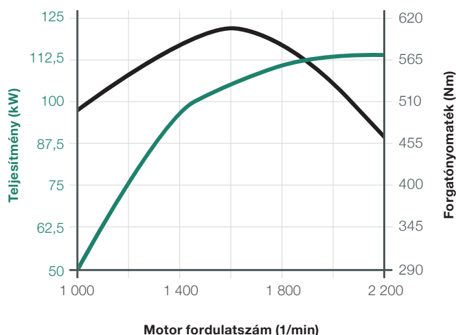
Deutz TCD 4.1 teljesítménygörbe (KT557, KT559)
