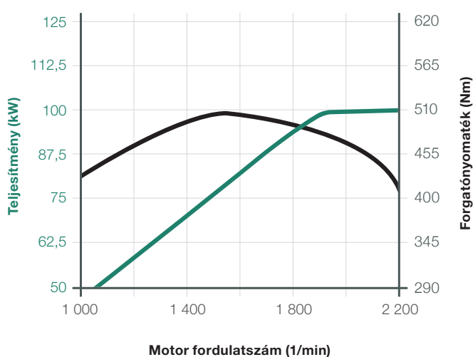
Deutz TCD 3.6 teljesítménygörbe (KT356, KT307, KT357, KT407, KT3610, KT457)
