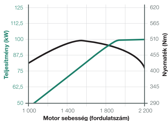
Deutz TCD 3.6 L4 (sorozat) teljesítménygörbéje
