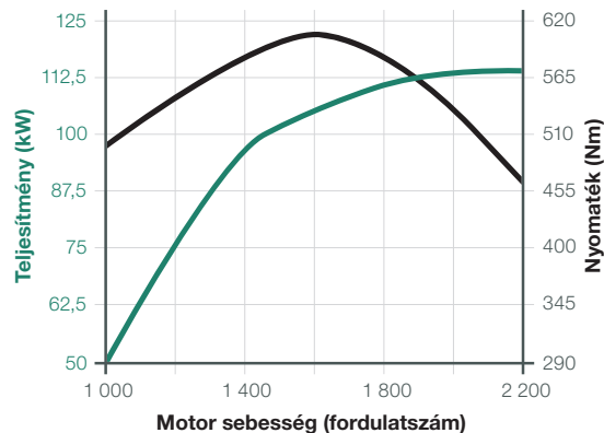
Deutz TCD 4.1 L4 (sorozat, opció) teljesítménygörbe
